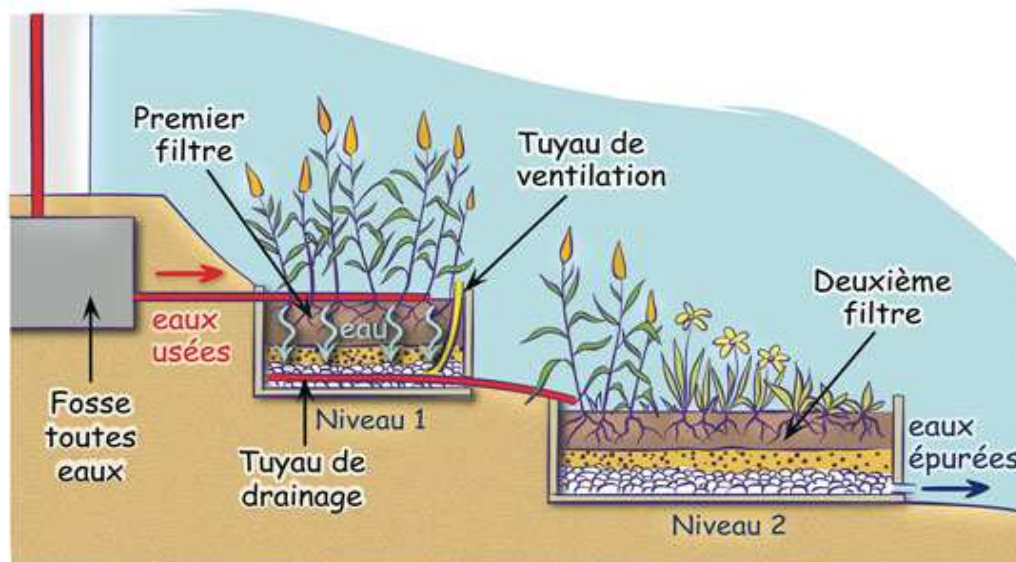
plan sommaire et fonctionnement d'une station par filtres à roseaux
